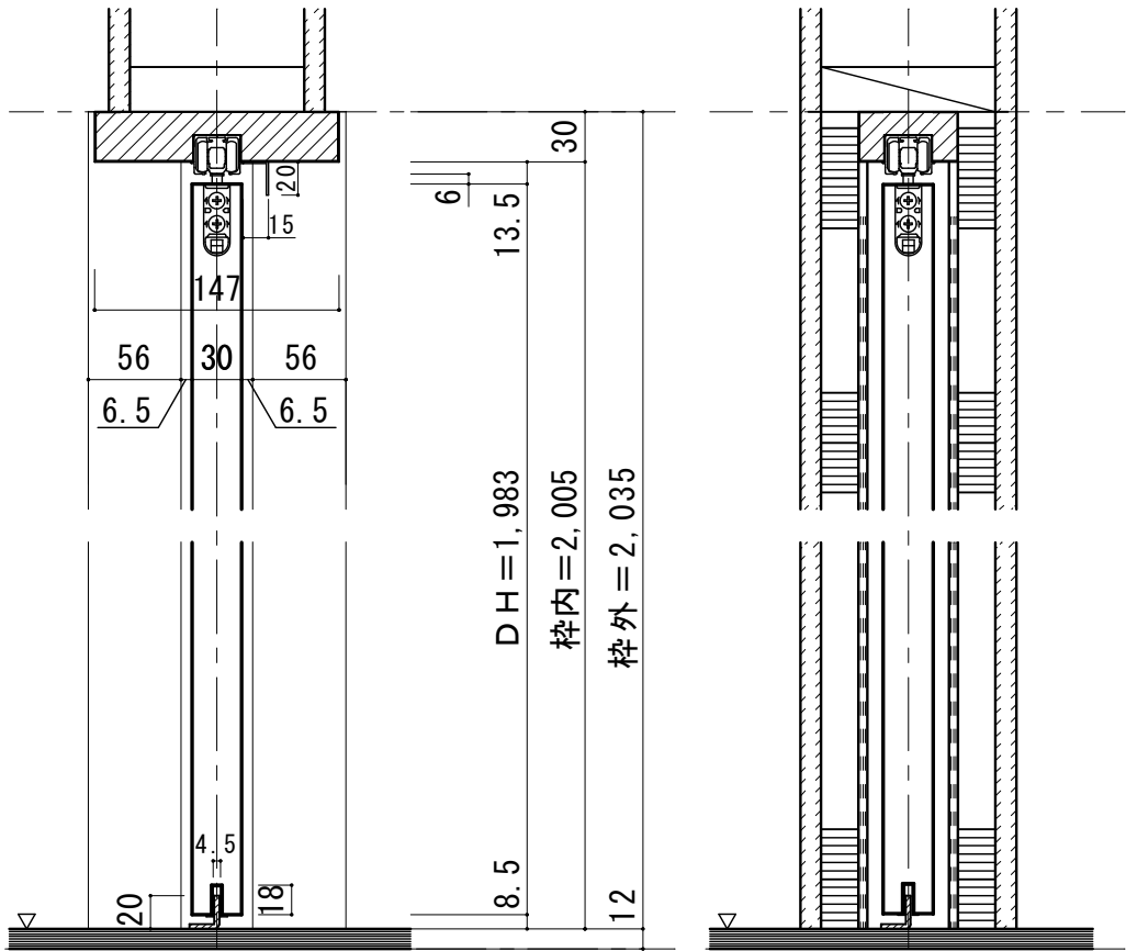
■縦断面図
