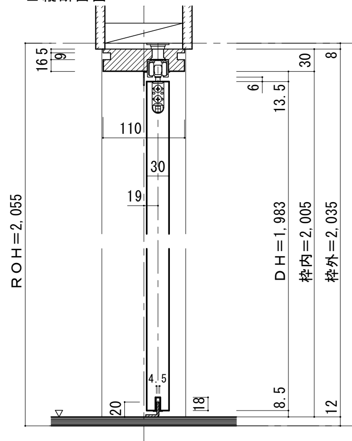
■縦断面図
