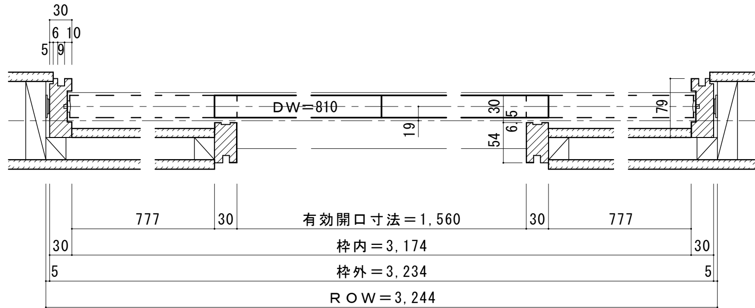
■横断面図
