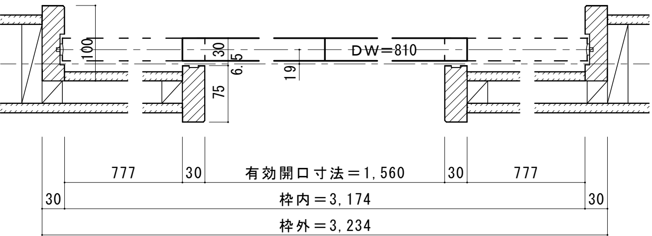
■横断面図
