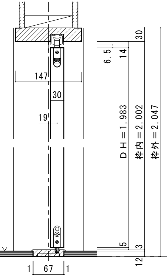
■縦断面図[敷居Q型]
