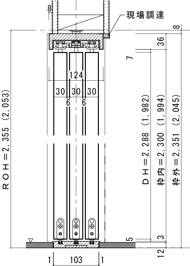
■縦断面図 H=8尺 (H=7尺)
