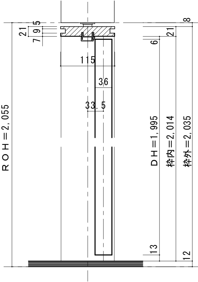
■縦断面図
