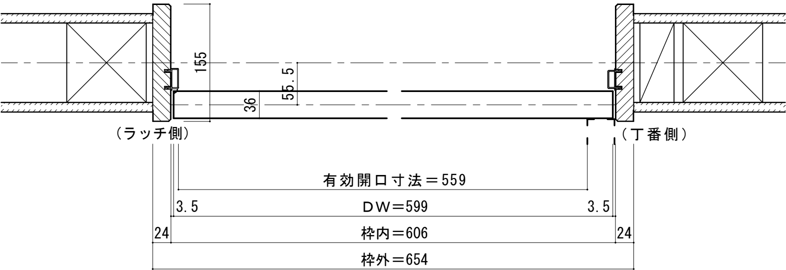
■ 横断面図 ※図示：右吊り元
