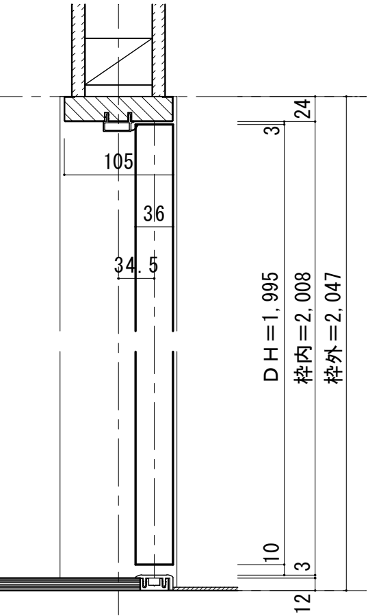
■ 縦断面図 [片ツハタイプ]
