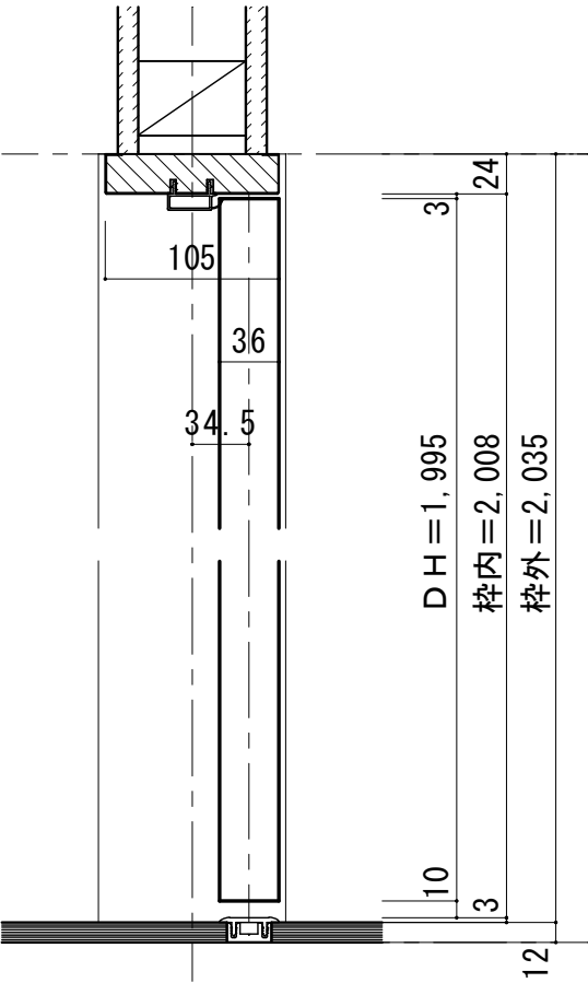
■ 縦断面図 [両ツハタイプ]
