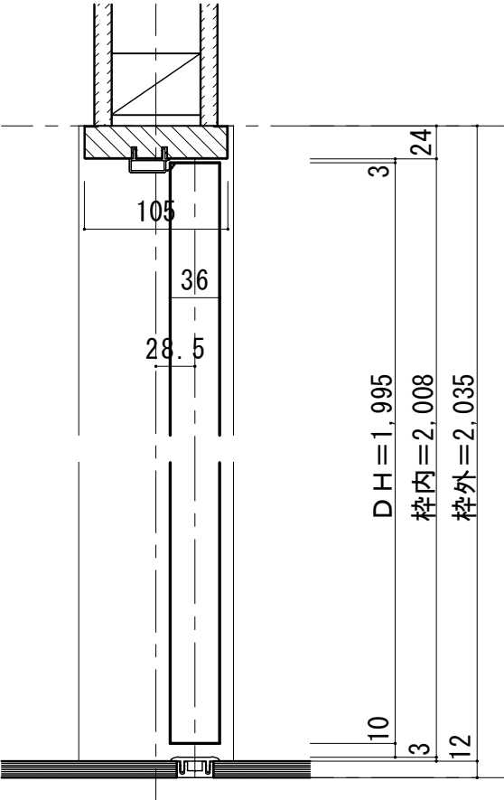
■ 縦断面図 [両ツハタイプ]
