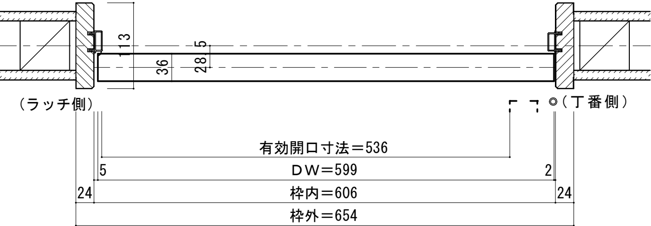
■ 横断面図
