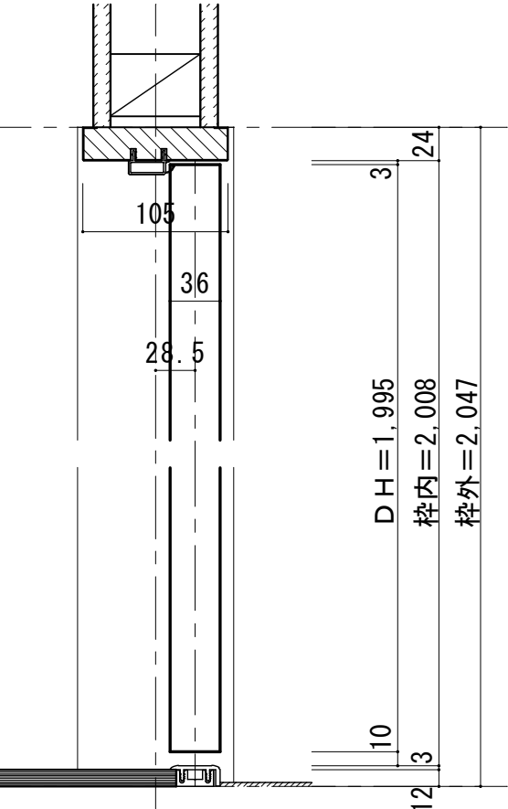
■ 縦断面図 [片ツハタイプ]
