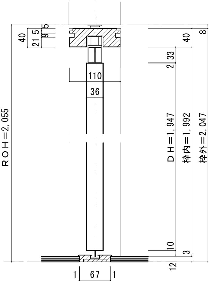
■縦断面図
