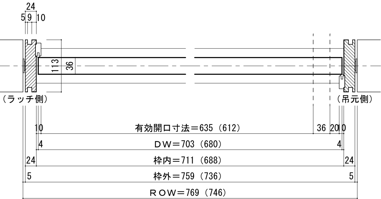
■横断面図 ※図示：右吊り元
