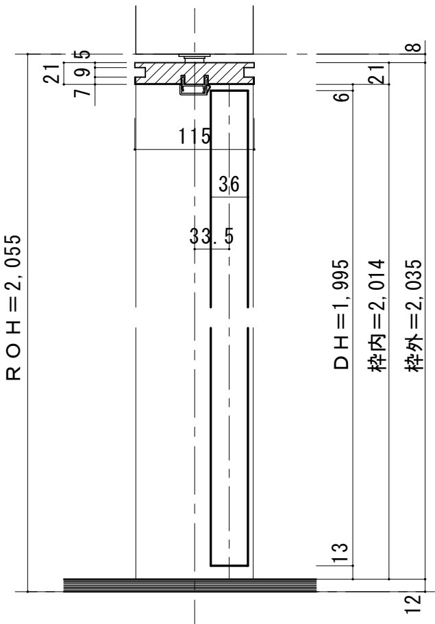
■縦断面図
