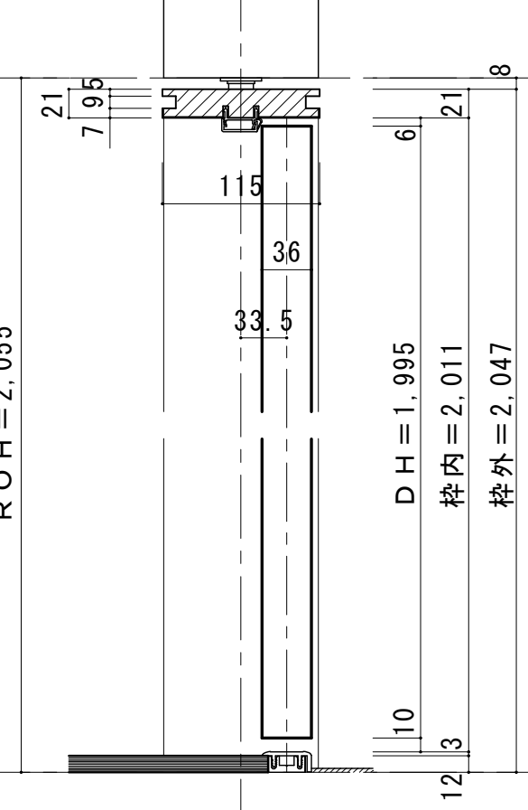
■縦断面図 [片ツパタイプ]
