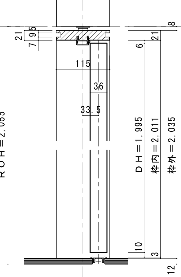
■縦断面図 [両ツパタイプ]
