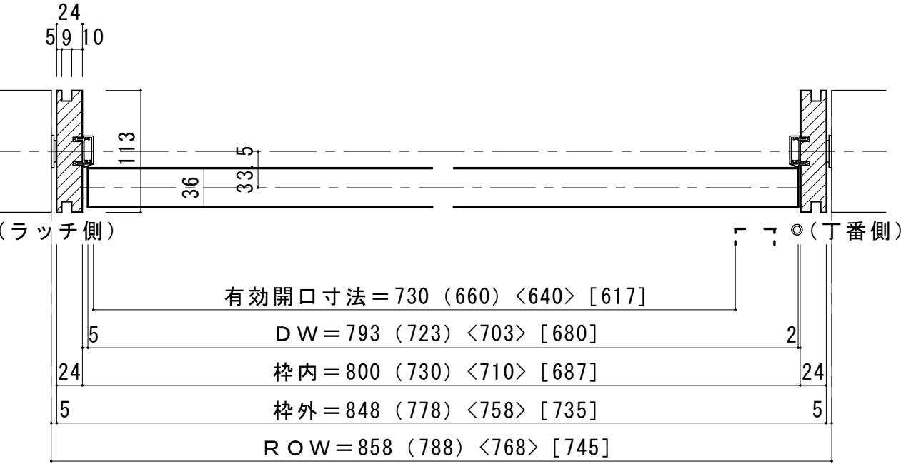
■横断面図 ※図示：右吊り元
