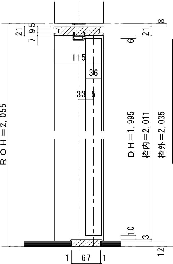
■縦断面図 [下枠Q型]
