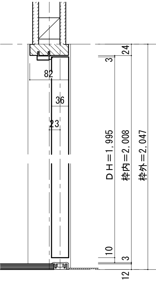
■ 縦断面図 [片ツハタイプ]
