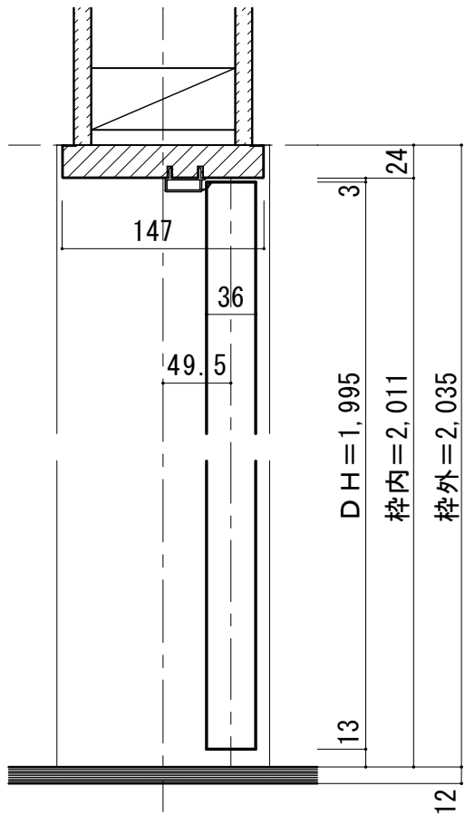
■ 縦断面図
