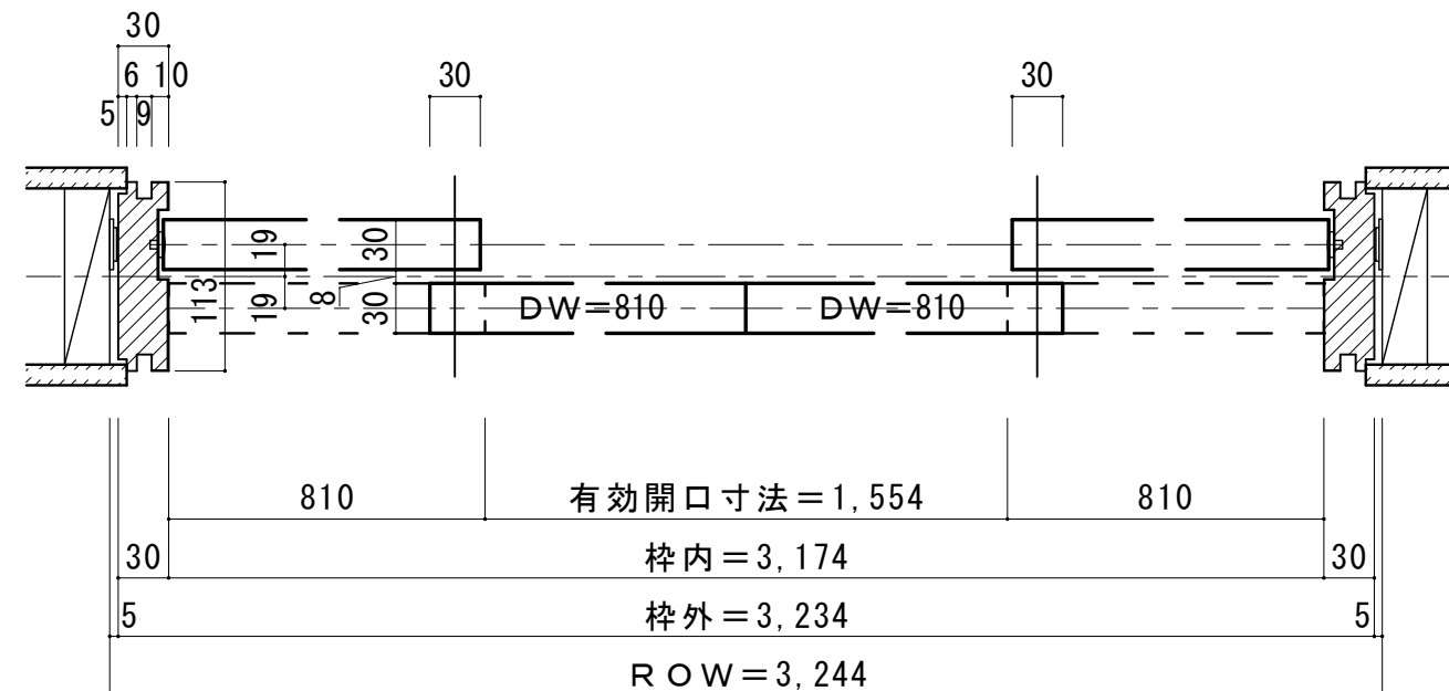
■横断面図
