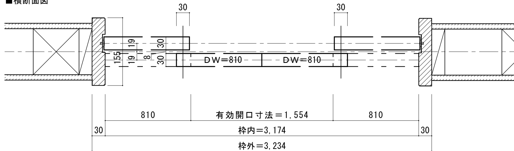
■横断面図
