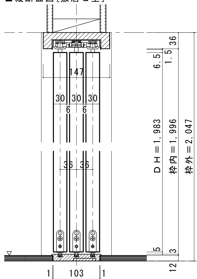
■縦断面図[敷居Q型]
