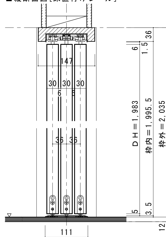
■縦断面図[床直付けレール]
