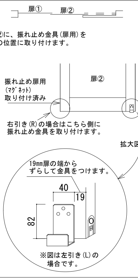
振れ止め金具 (扉付け用) 取り付け
