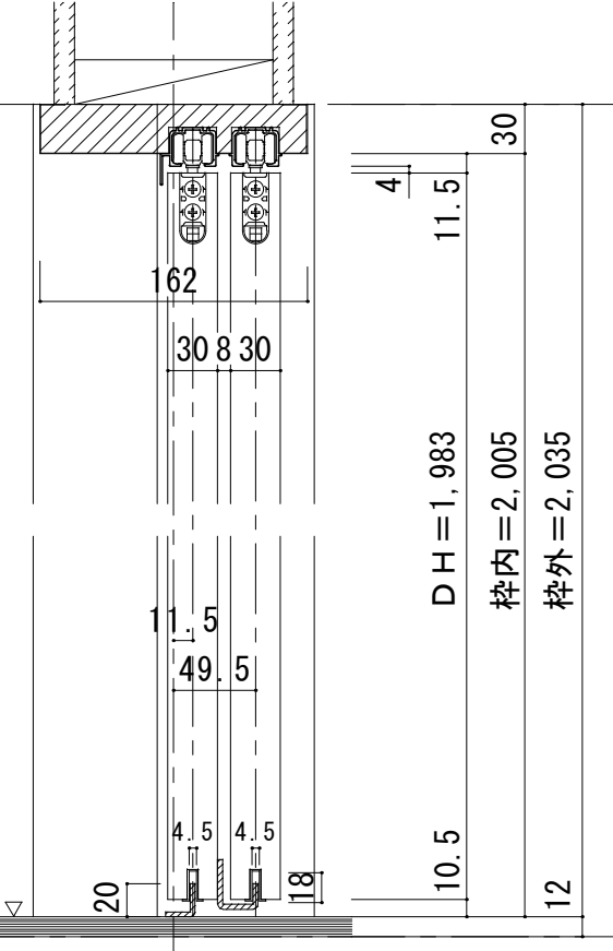
■縦断面図
