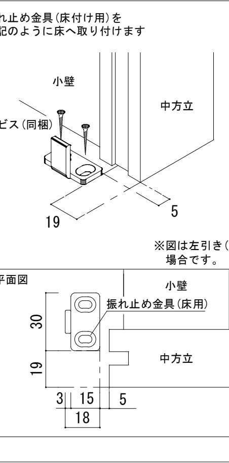
振れ止め金具 (床付け用) 取り付け
