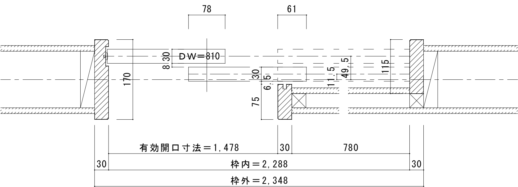
■横断面図 ※図示：左引き手
