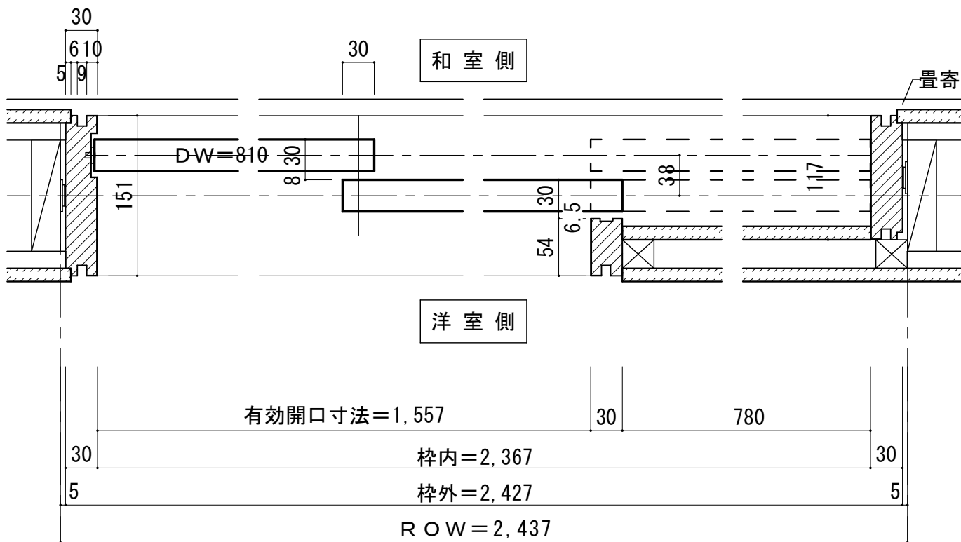
■横断面図 ※図示：左引き手
