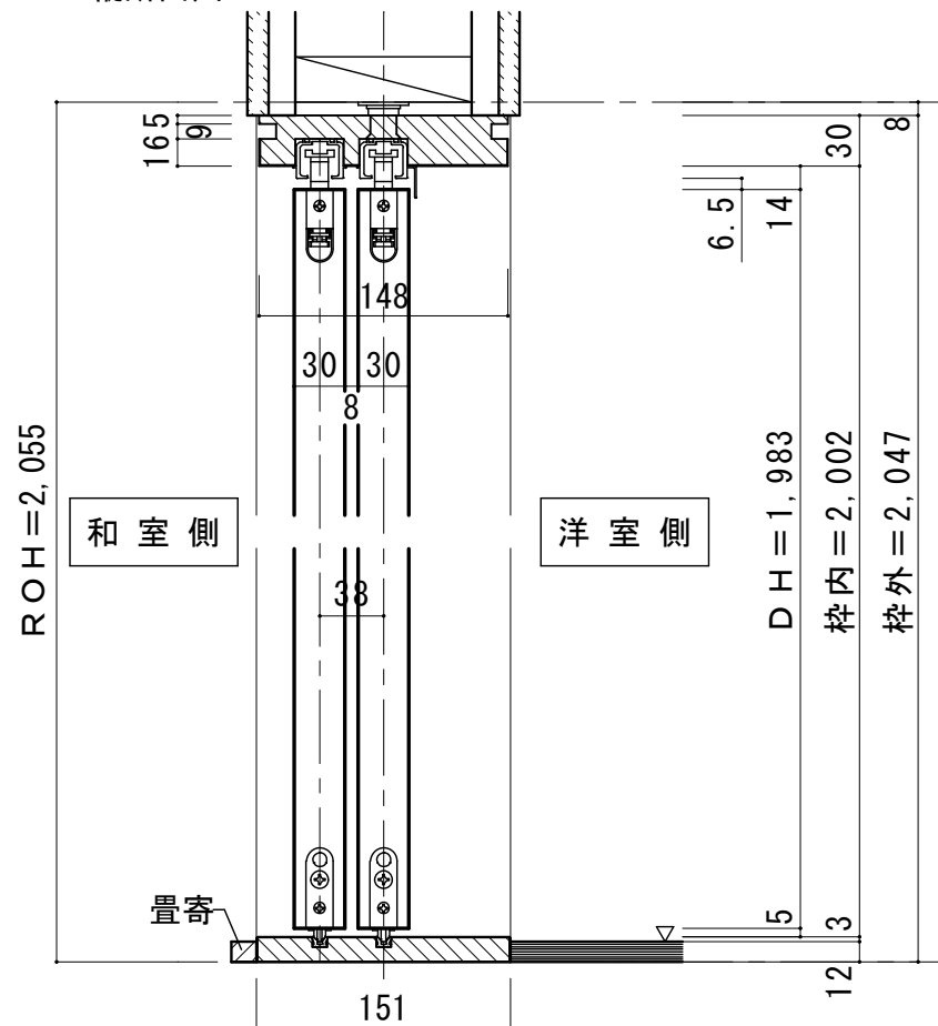
■縦断面図
