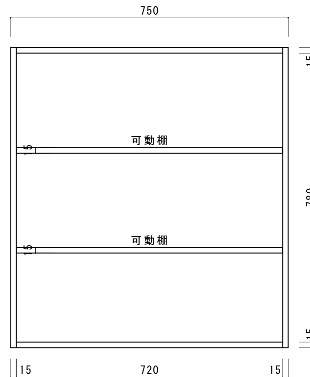
正面図
