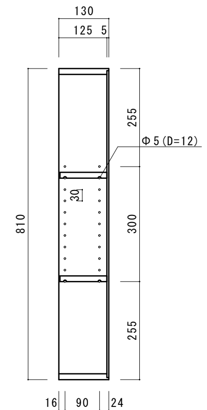
断面図
