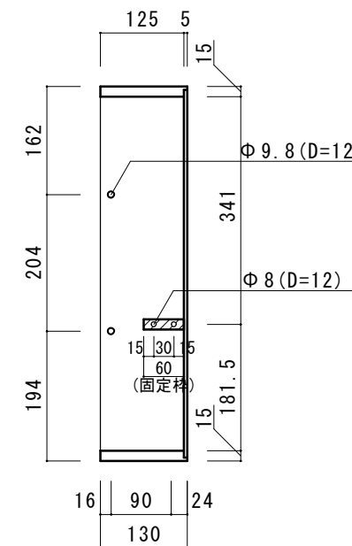
断面図
