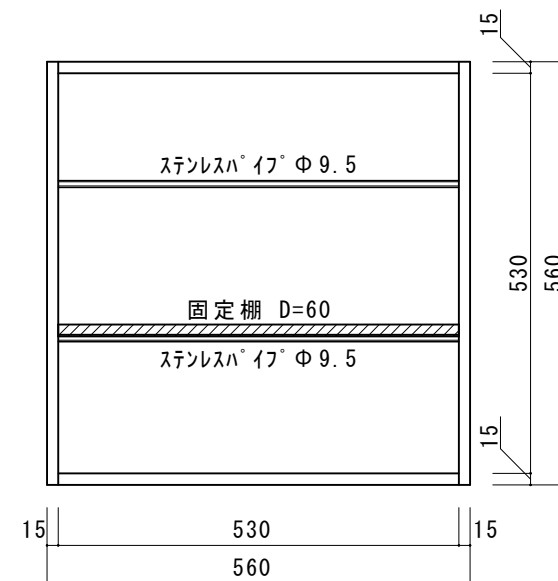
正面図
