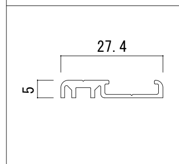
床直付けレール詳細図 (S=1/1)
