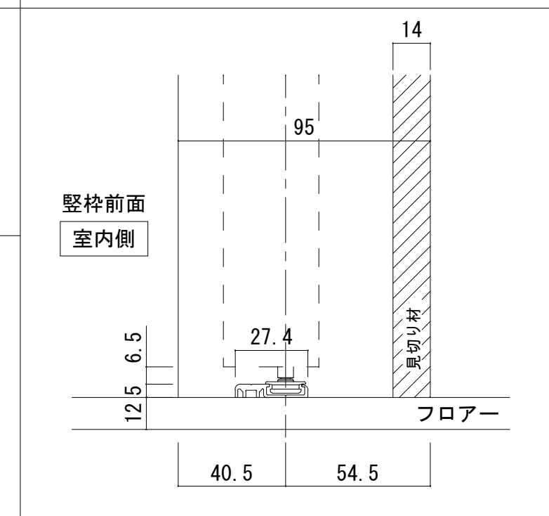
床直付けレール取り付け位置 (S=1/2)
