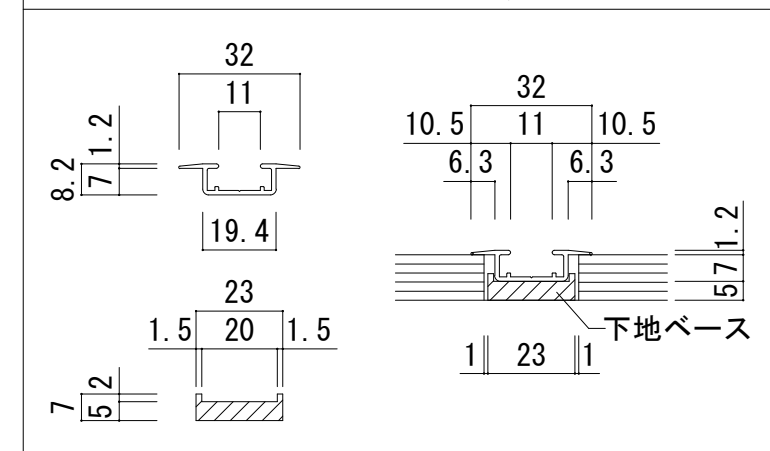
■ レール拡大図 (S=1/2)
