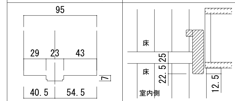
■ レール拡大図 (S=1/2)
