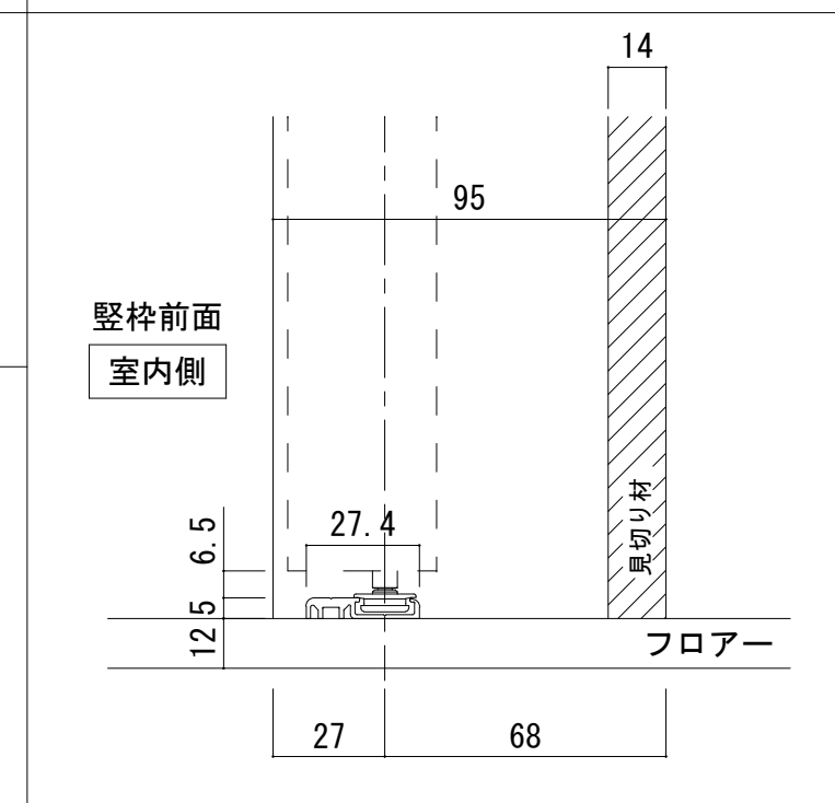
床直付けレール取り付け位置 (S=1/2)
