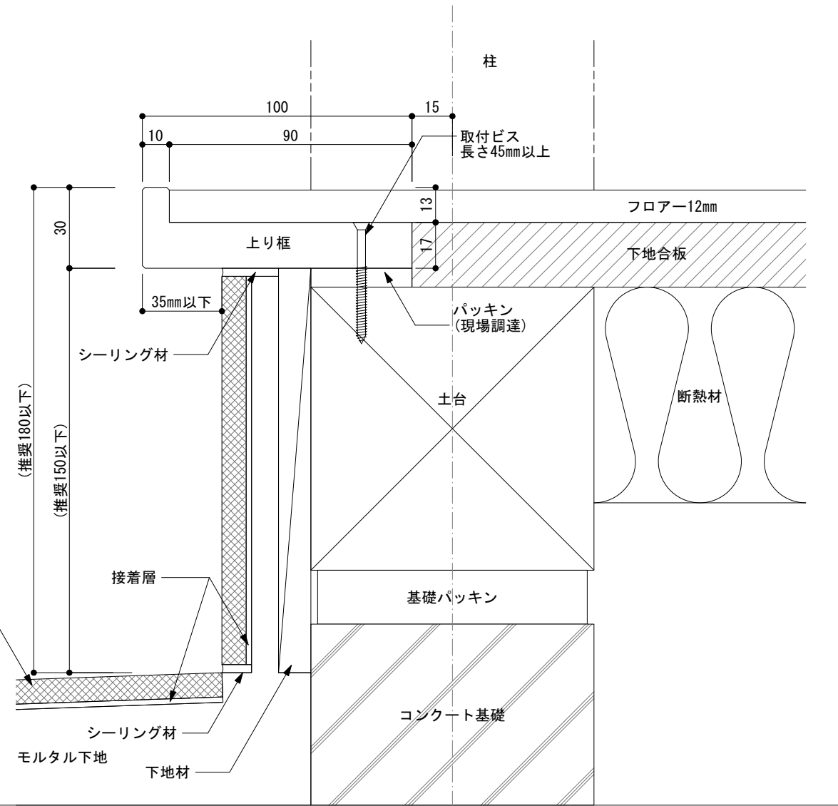
参考納まり図
