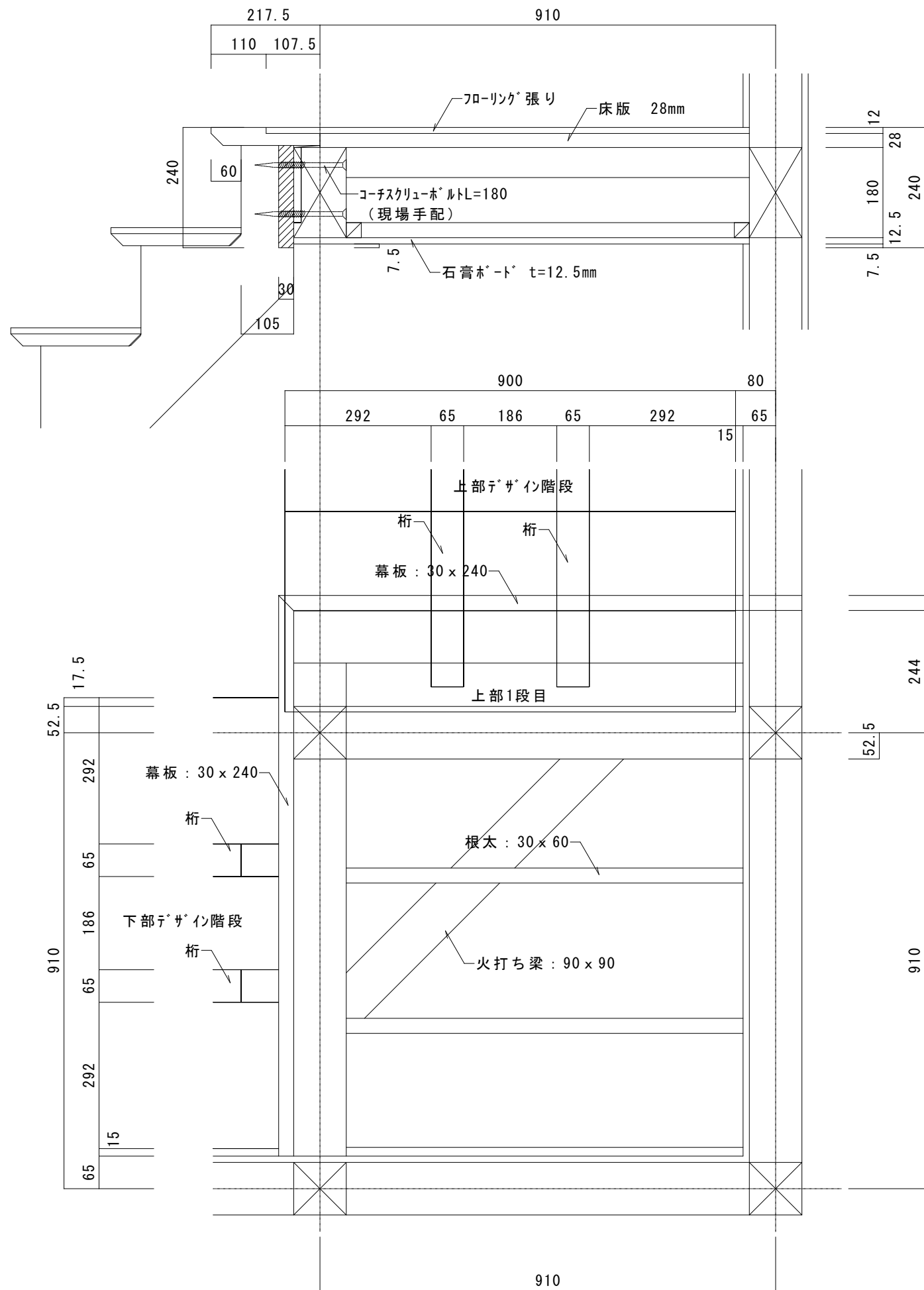
【踊り場詳細図（幕板納まり）】
