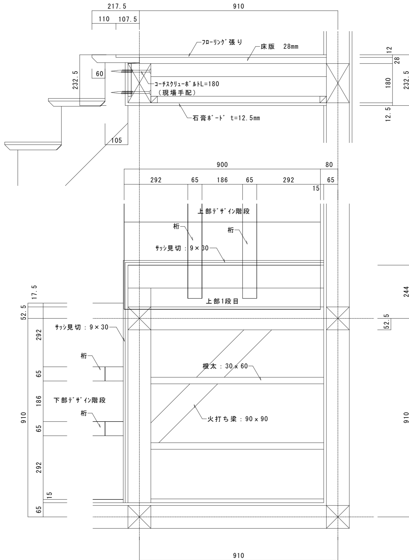
【踊り場詳細図（クロス巻き込み納め）】
