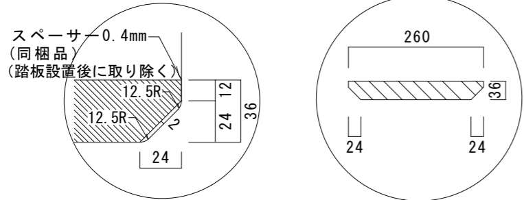
A部拡大図 S=1:30
