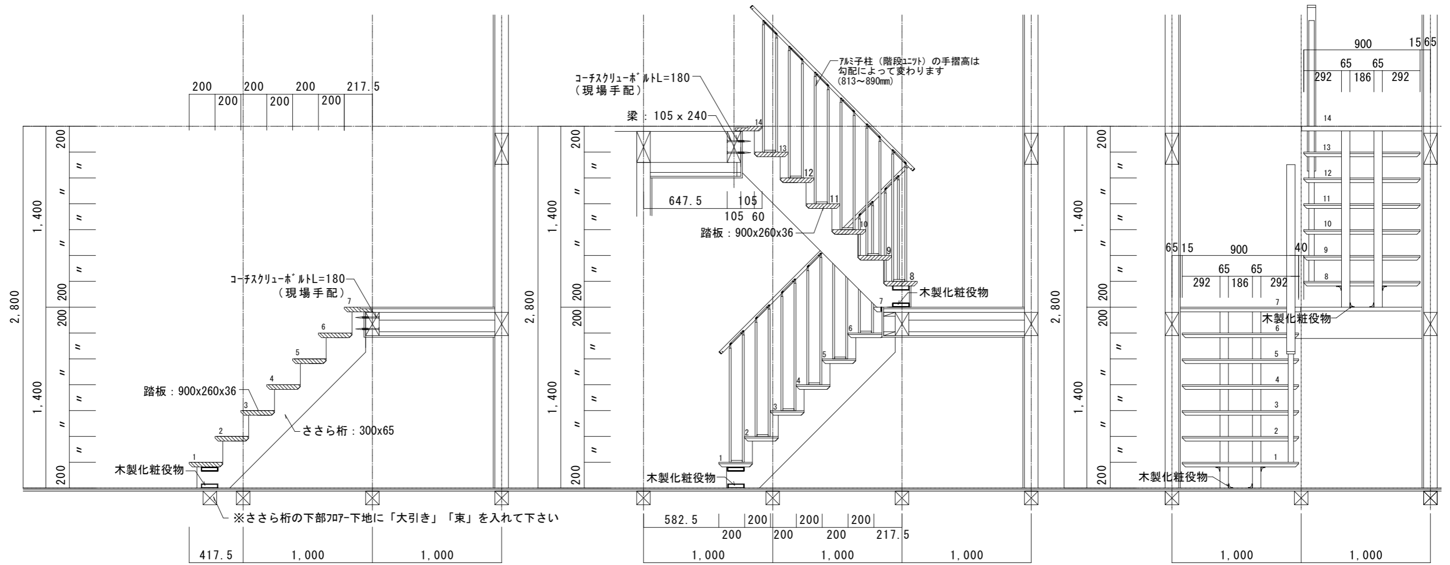
階段断面図 A S=1:30
