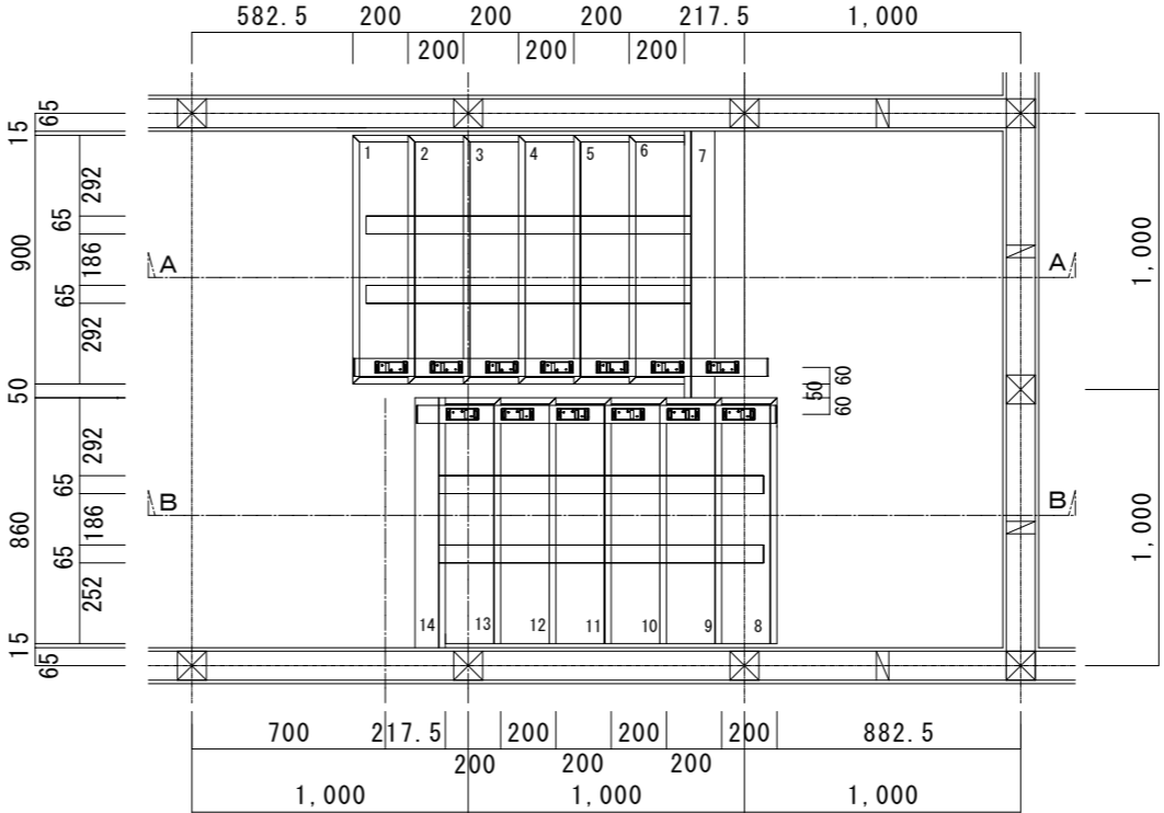
階段平面図 S=1:30
