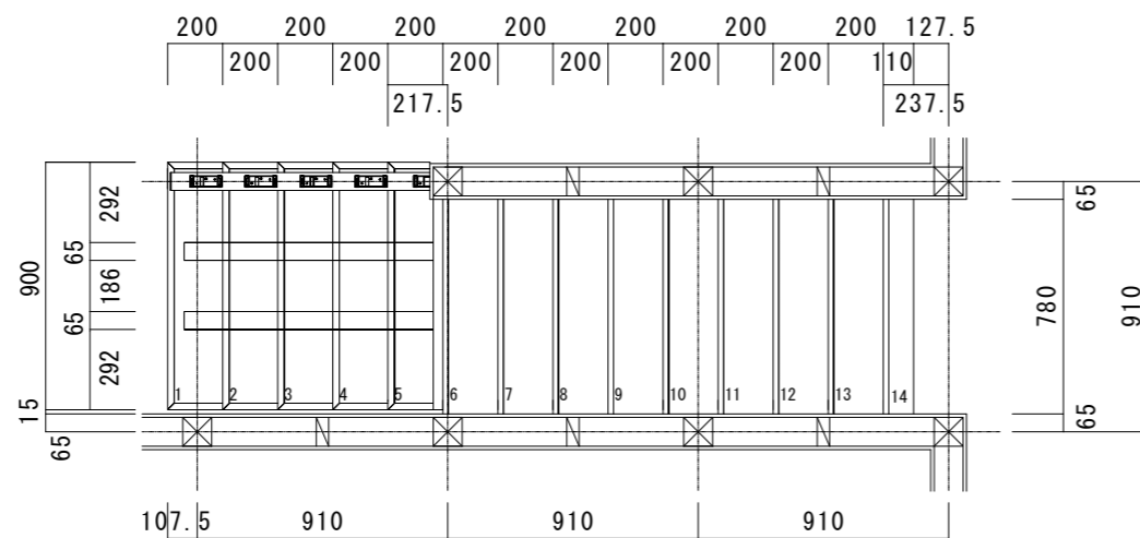
階段平面図 S=1:30
