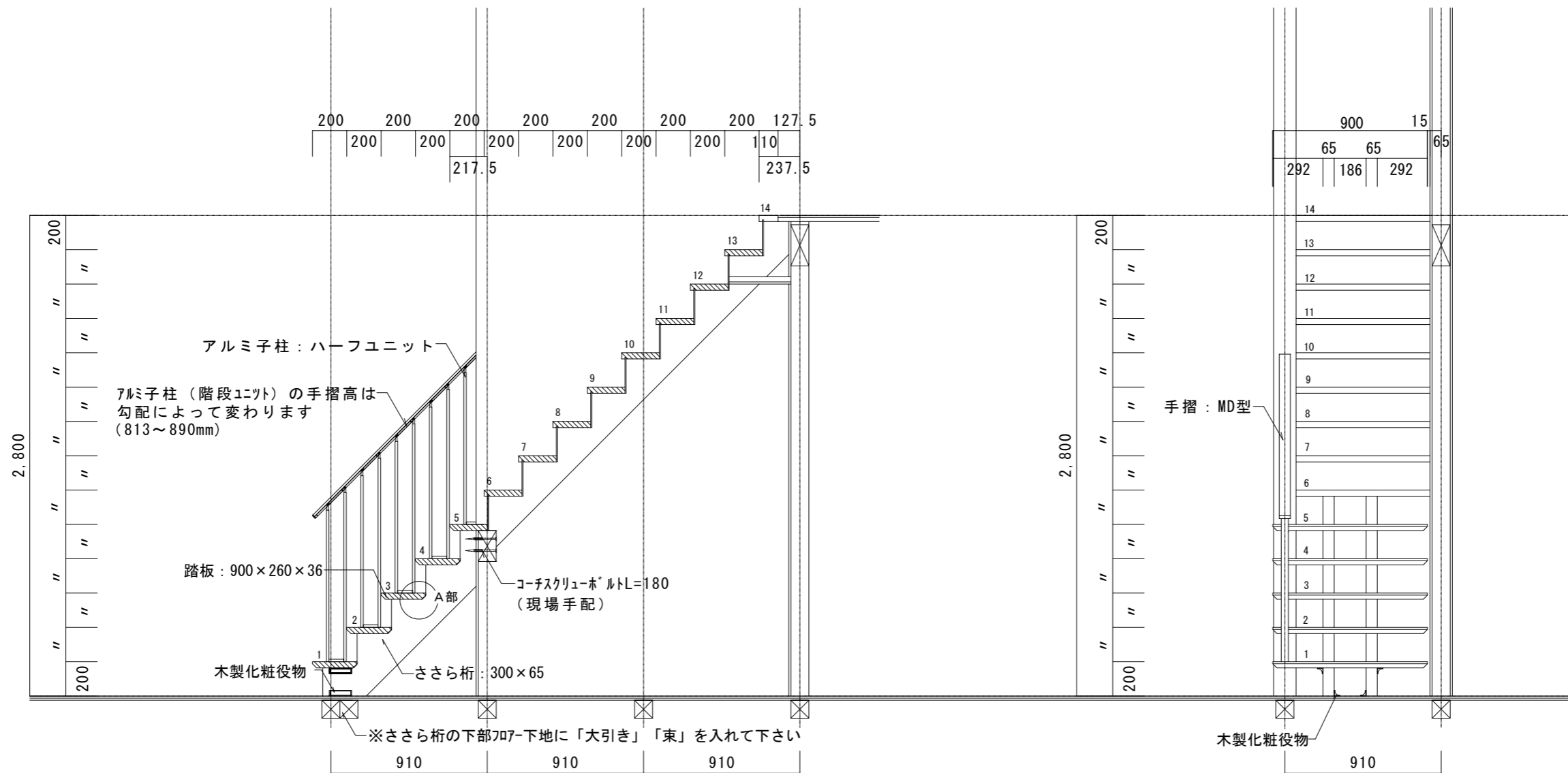
階段断面図 S=1:30
