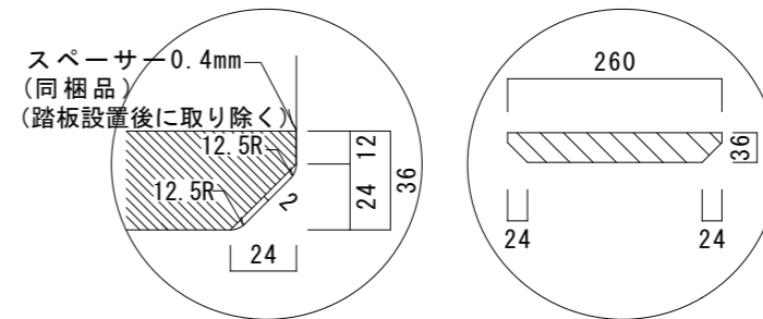
A部拡大図 S=1:30
