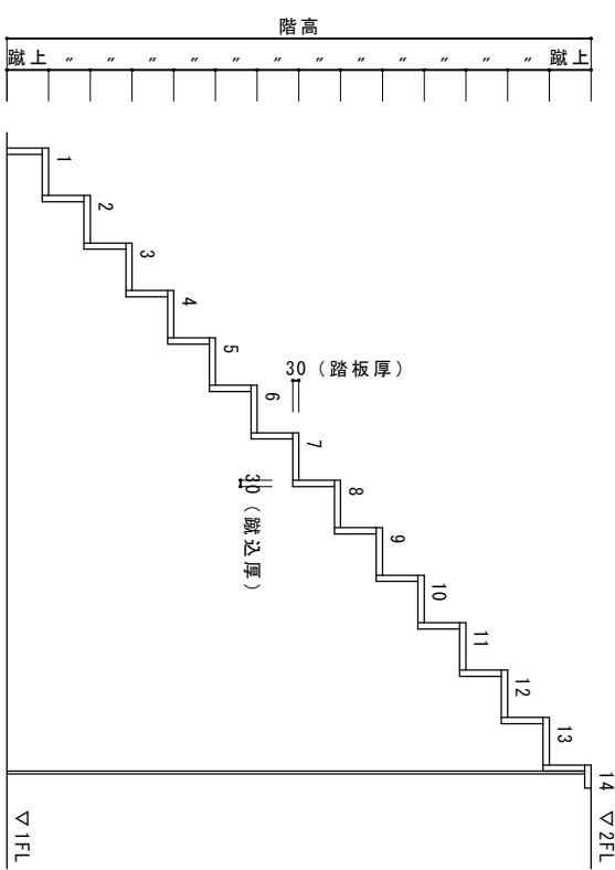
A-A断面図
