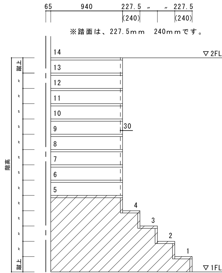
B-B断面図
