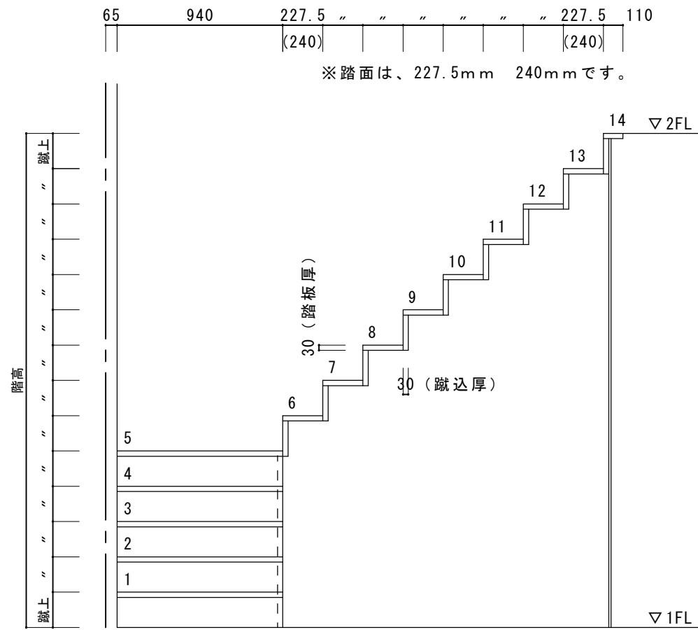
A-A断面図
