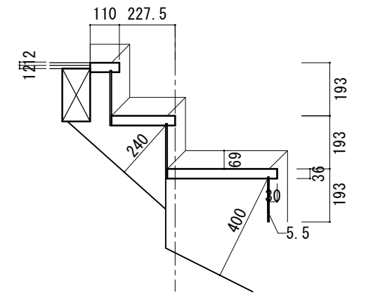
b 部廻り直接続部納まり図 S=1/20
