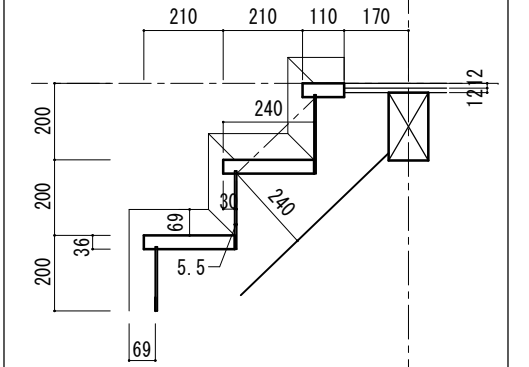
c 部廻り直接続部納まり図 S=1/20
