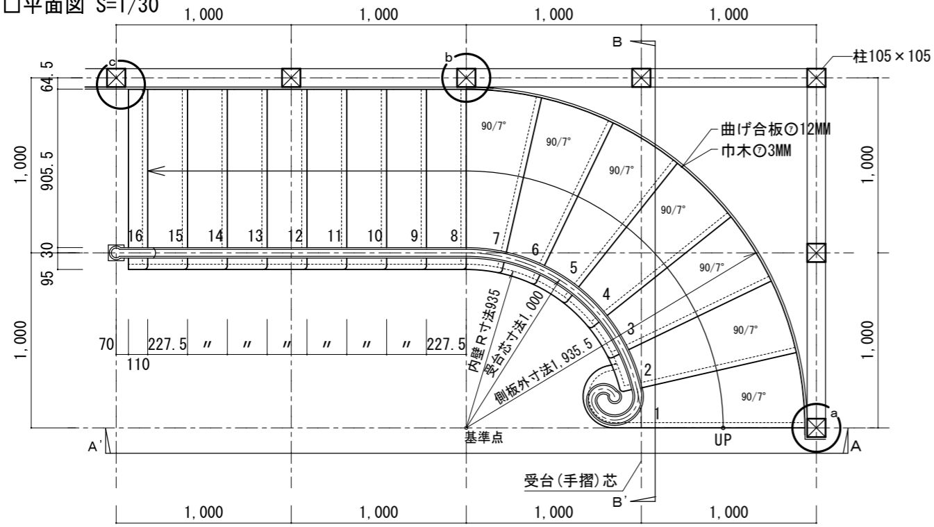
□平面図 S=1/30
