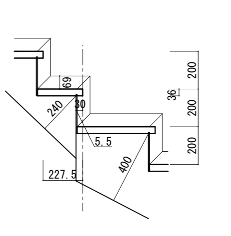
b 部廻り直接続部納まり図 S=1/20
