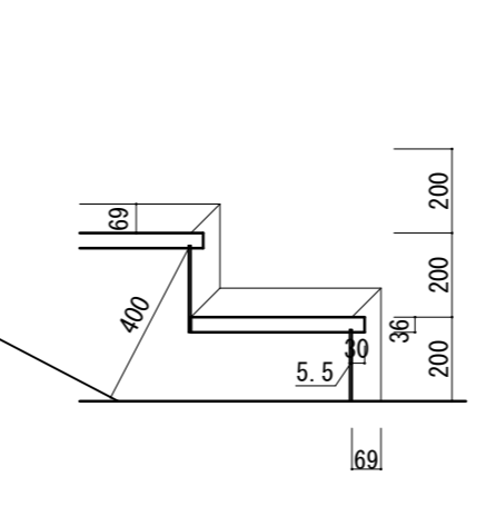
a 部階段下部納まり図 S=1/20
