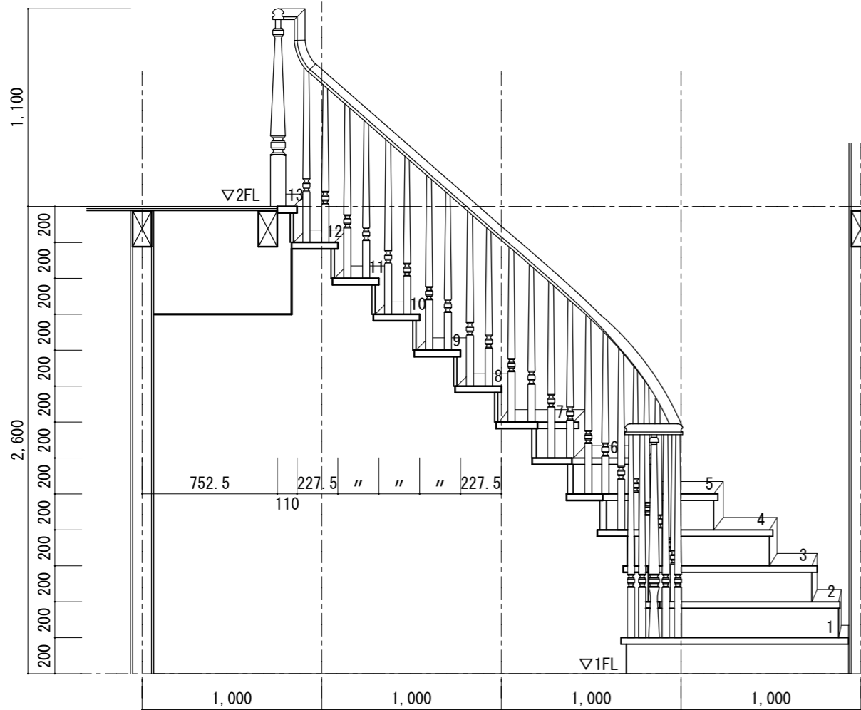
□断面図 A-A' S=1/30
