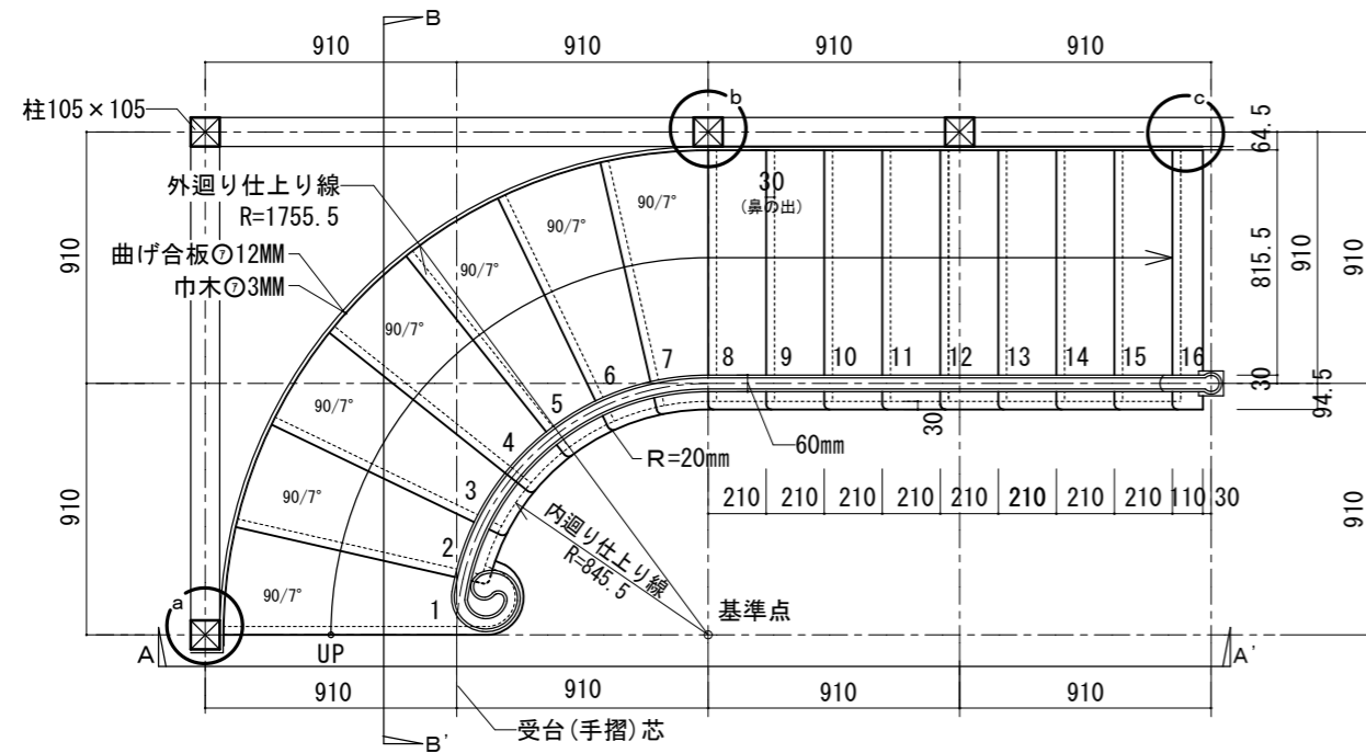
□平面図 S=1/30
