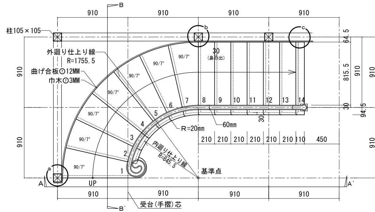
□平面図 S=1/30
