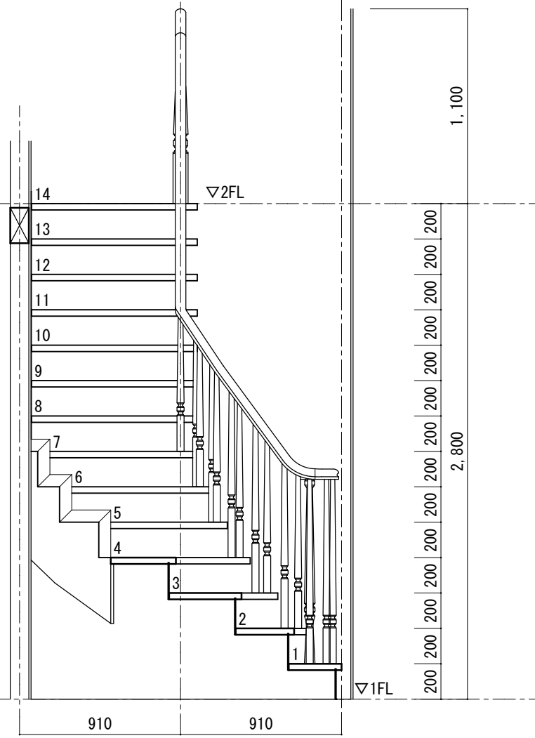
□断面図 B-B' S=1/30
