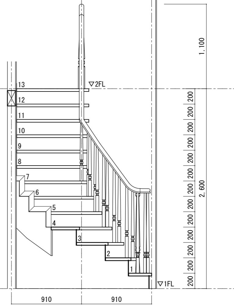
□断面図 B-B' S=1/30
