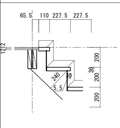
c 部廻り直接続部納まり図 S=1/20
