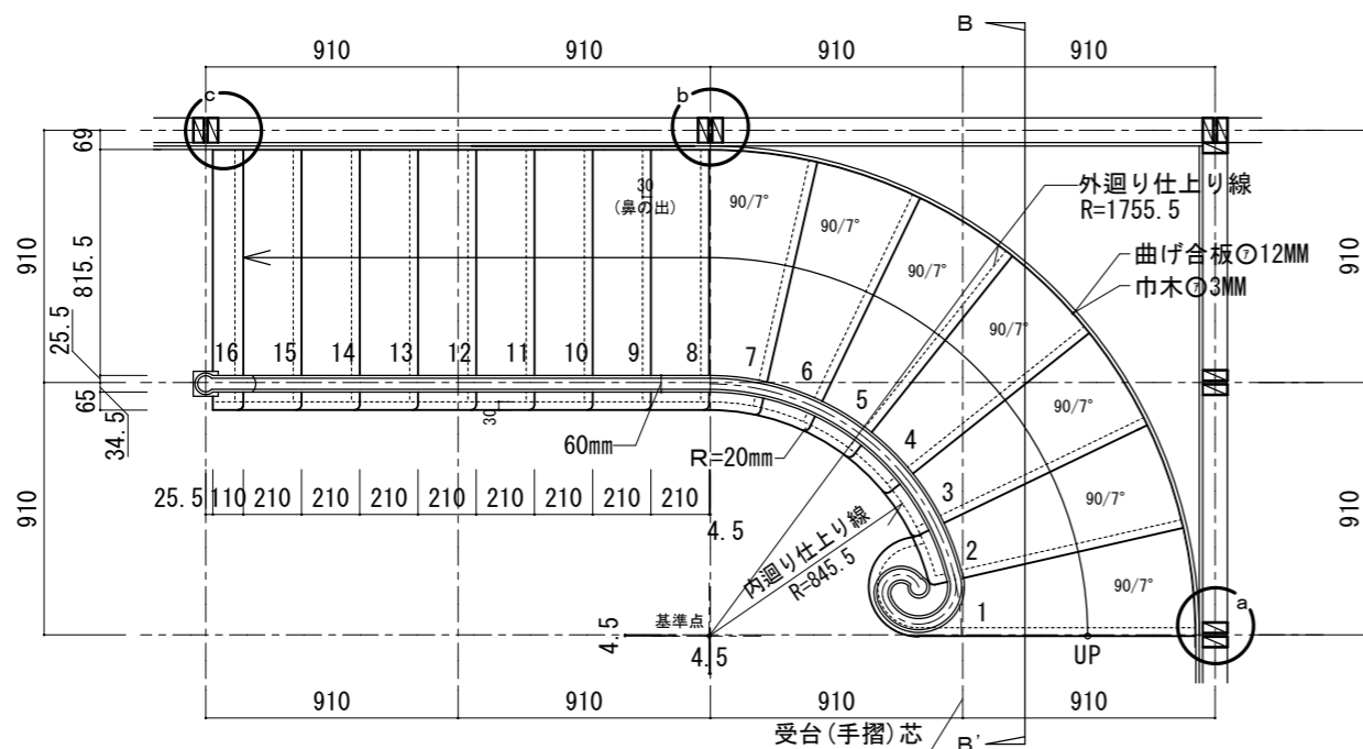
□平面図 S=1/30
