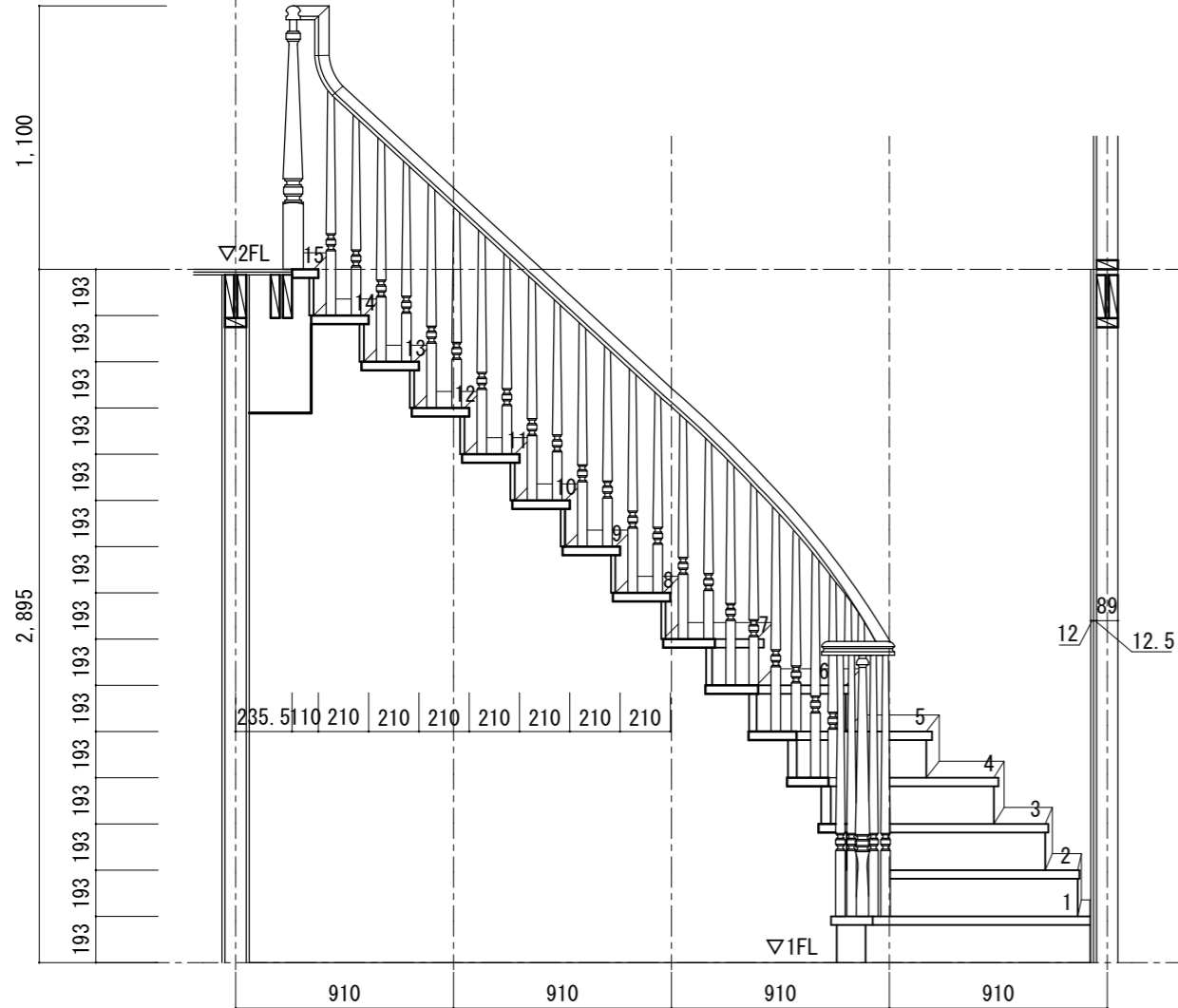
□断面図 A-A' S=1/30
