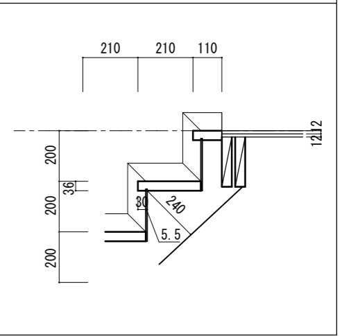
c 部廻り直接続部納まり図 S=1/20
