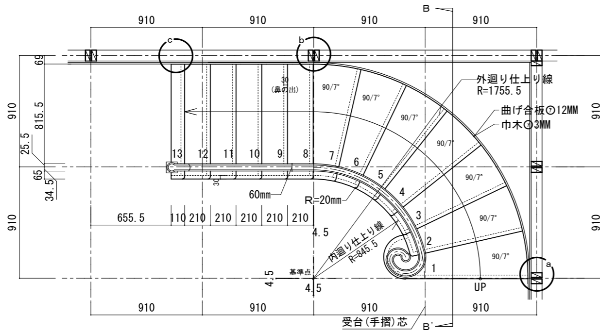
□平面図 S=1/30
