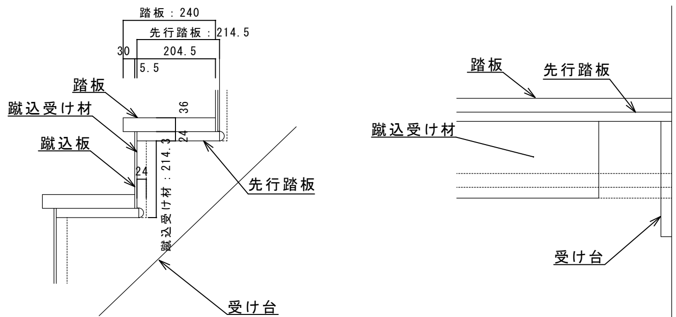
階段 受け台部分詳細図 SCL=1/10
