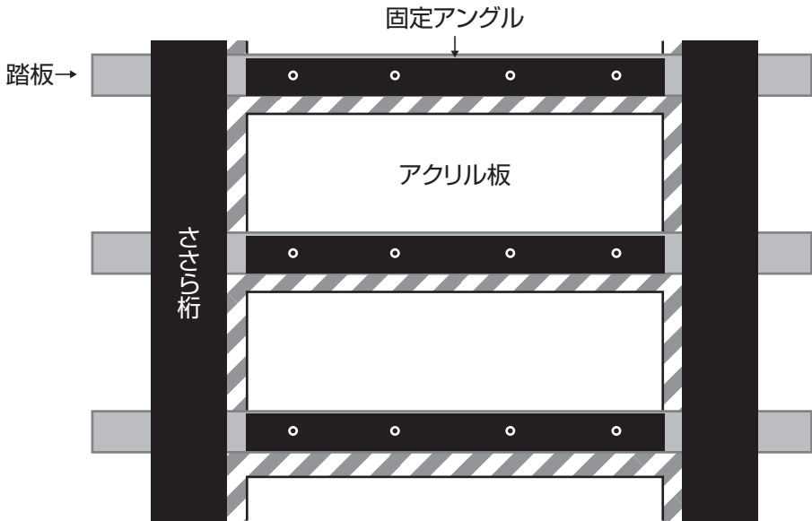
デザイン階段Light全体図(アクリル蹴込パネル施工時)
