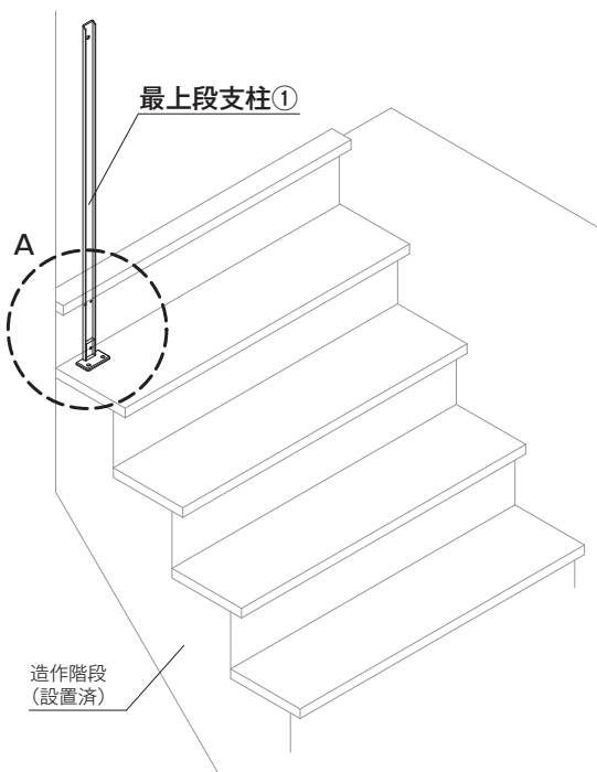
最上段支柱の取付
