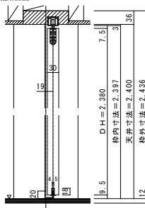
■縦断面図
