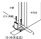
振れ止め金具(床付用)取り付け
