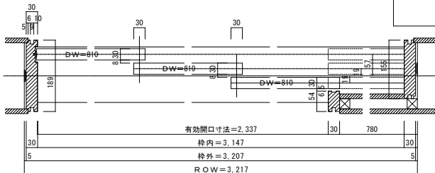
■横断面図
